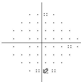
Desvio Padrão
