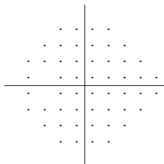
Desvio Total
